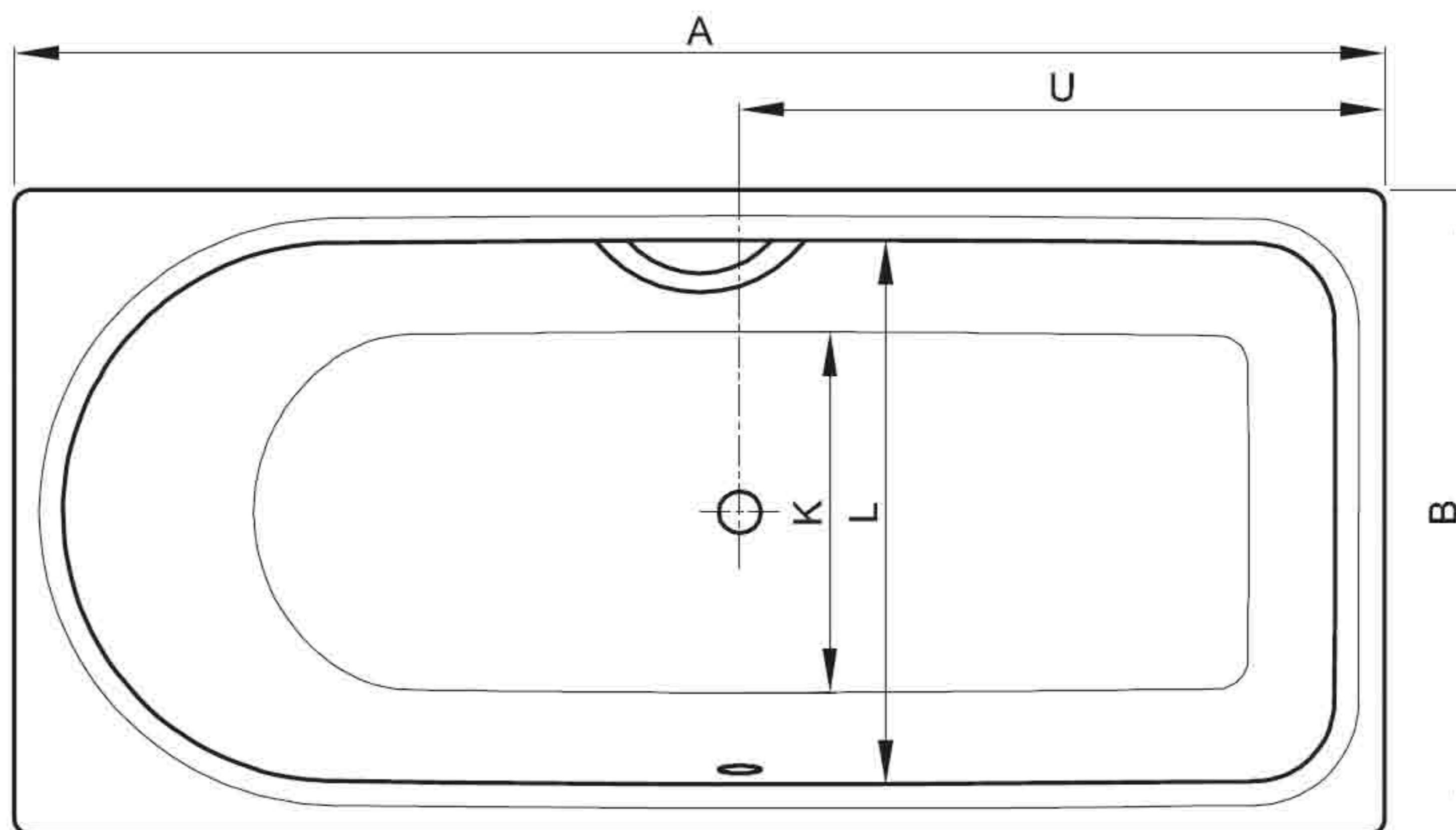
Výkres 170 x 80 cm, strana nohou vpravo, přepad vpředu, obj. č.: 8851, 8853, 8855, 8865, 8857
