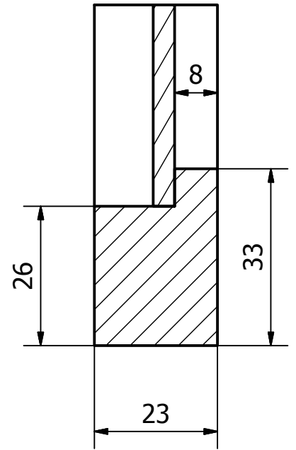
A-A ( 1 : 1 )
