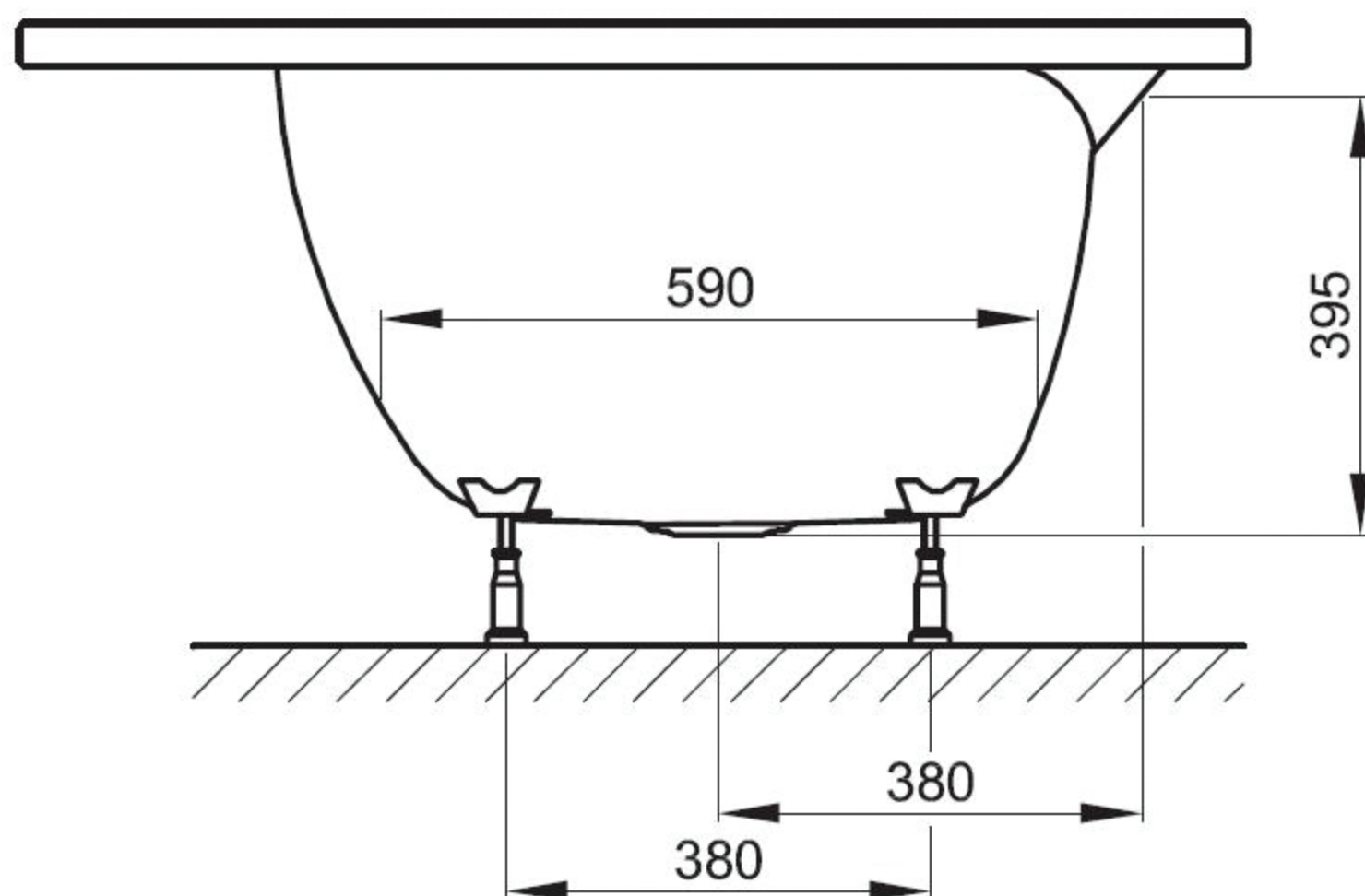
Výkres: Levé provedení, obj. č. 6052
