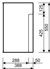
Obudowa frontowa
