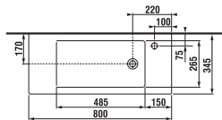
Umyvadlo 80 cm
