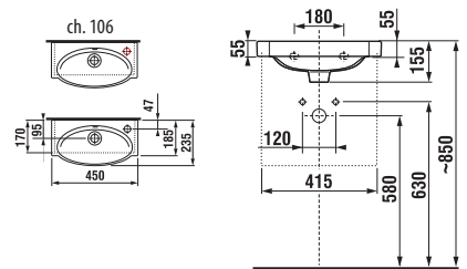
Skříňka s umývatkem 45 cm
