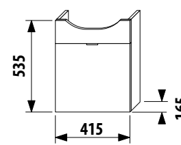
Skříňka s umývatkem 45 cm
