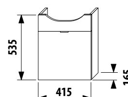
Skříňka s umývatkem 45 cm
